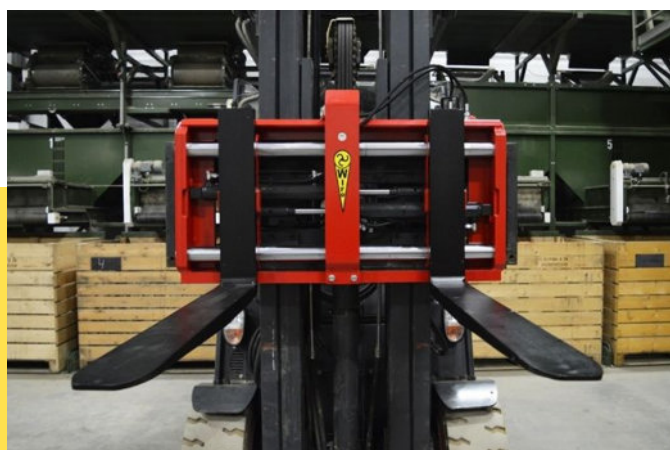
Vorkenversteller VV25
