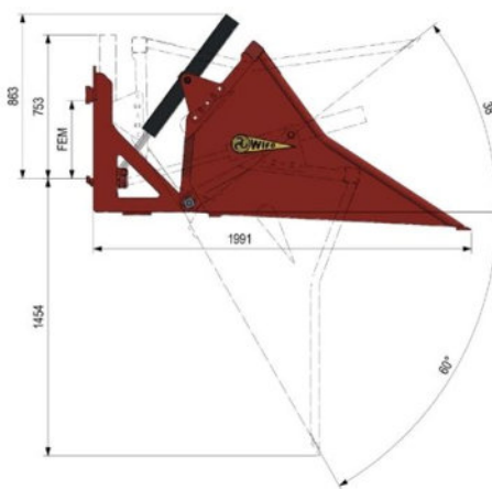
WIFO aardappelschapbak op vorkenbord
