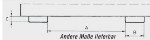
Einfahrtaschen-Innenmaße (mm)
